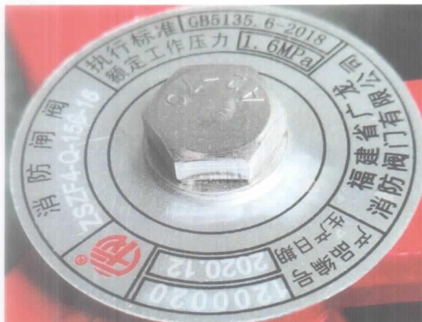
消防闸阀 ZSZF4-Q-150-16
