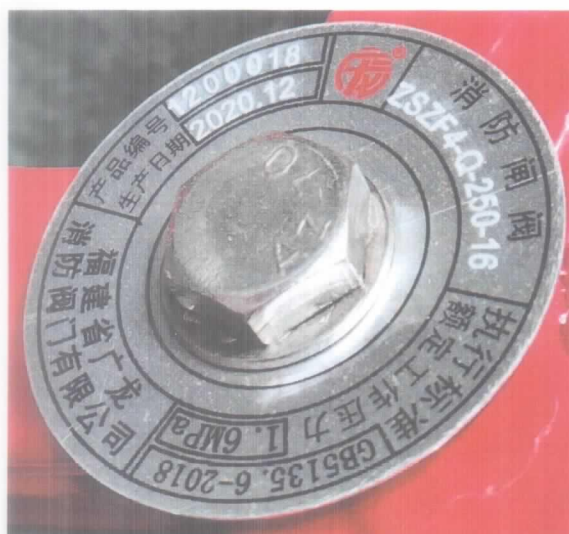
消防闸阀 ZSZF4-Q-250-16
